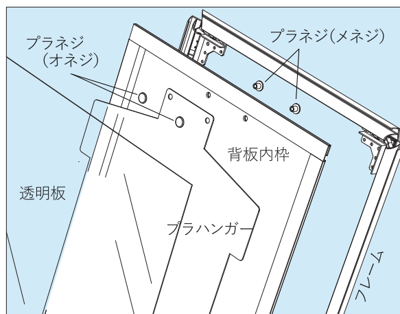
ユニフォーム額 L・M サイズの構造 (フレームサイズは異なる)
