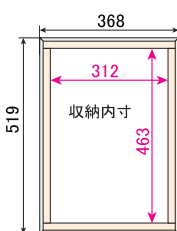
立体額 S サイズ
