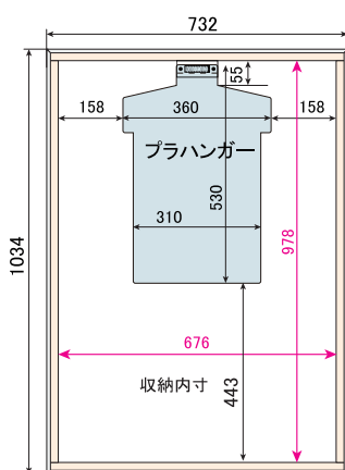
立体額 L サイズ
