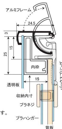
ユニフォーム額 (L・M)
