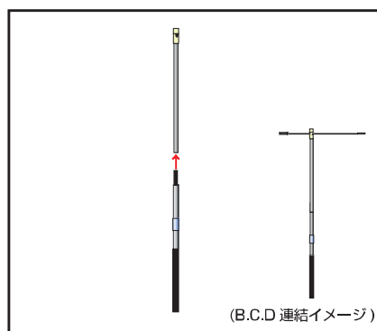
①テンションバー C.D 種を連結する。
