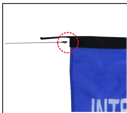
②メディア袋加工部分に連結したテンションバーを通す。
