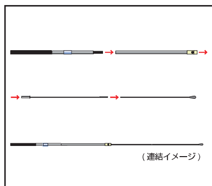
①テンションバー 4 種を連結する。
