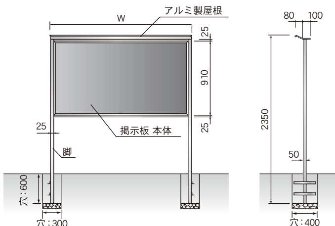
K C型屋外掲示板
