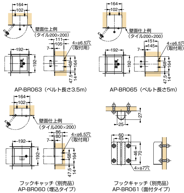
フックキャッチ (別売品)
