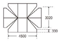
天幕(平面図)
