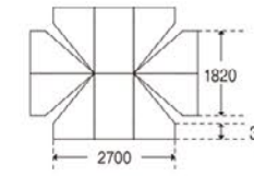
天幕(平面図)
