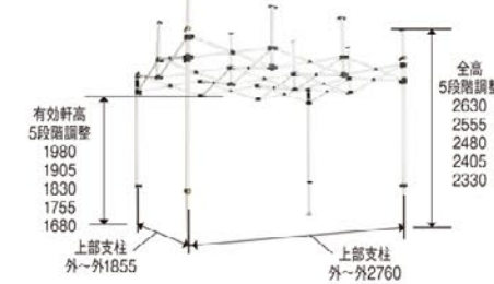
フレーム
