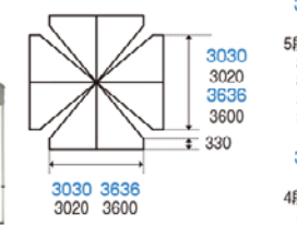
天幕(平面図)
