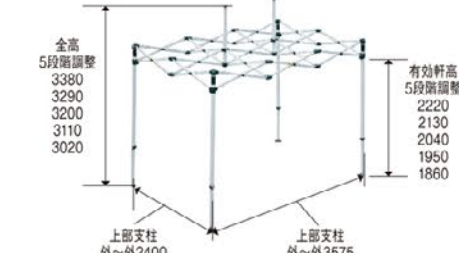
フレーム
