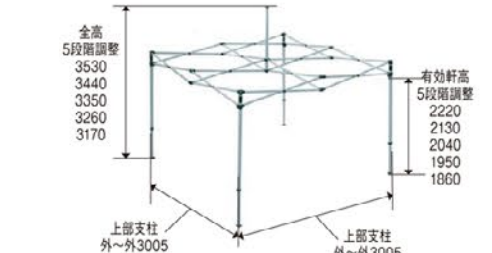
フレーム
