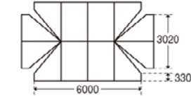
天幕(平面図)
