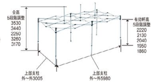
フレーム
