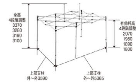
フレーム
