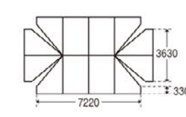
天幕(平面図)
