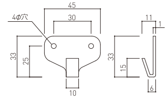
SK-FC-3 ¥530 材質: ステンレス (SUS304)
