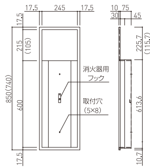
※ ( ) 寸法はSK-FEB-52
