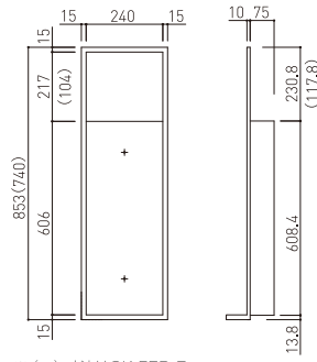
※ ( ) 寸法はSK-FEB-5
