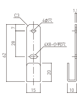
SK-FC-2 ¥380 材質: フック金具/SPCC (ユニクロメッキ)
