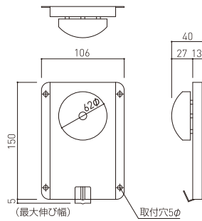
SK-FB-1 ¥12,600 材質: カバー/ステンレス (SUS304)
