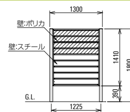
立面図
