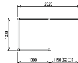
平面図
