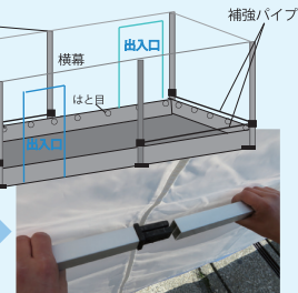
SNWT-3060連結使用例
