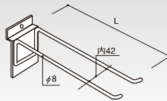
(P-大) クロームメッキ ダブルフック HP-WHK-200 L(mm) コードNo. 定 価 重さ(g) 200 55091 ¥1,890 274 250 55092 ¥2,250 313 300 55093 ¥2,610 354 梱30
