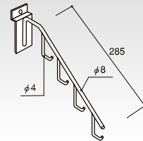
(P-中) クロームメッキ 袋物フック HP-FHK コードNo. 定 価 55132 ¥2,920 梱30 242g
