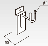
(P-小) クロームメッキ ネクタイフック HP-NTHK コードNo. 定 価 55101 ¥1,200 梱50 51g
