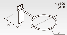
(P-小) クロームメッキ リングフック HP-100 RHK 内φ(mm) コードNo. 定 価 重さ(g) 100 55111 ¥2,700 137 150 55112 ¥2,920 173 梱50
