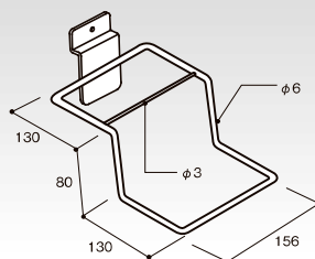
(P-U新) クロームメッキ シューズフック(2段) HP-SWHK コードNo. 定 価 55139 ¥1,950 梱15 285g
