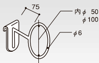
(P-大) クロームメッキ 垂直リングフック HL-V50RHK コードNo. 定 価 重(g) 50 62083 ¥2,250 106 100 62084 ¥2,620 140 棚30
