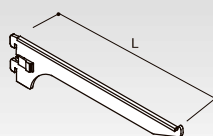
ツメ付ブラケット 2爪(SP) クロームメッキ NX12-150 SP L(mm) コードNo. 定 価 重さ(g) 150 81502 ¥360 100 200 81504 ¥400 120 250 81507 ¥450 150 ※ブラケット用サポートが必要です。
