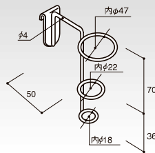
(P-大) クロームメッキ リングフック 3連 HL-R3HK コードNo. 定 価 重(g) 93g 62081 ¥3,450 棚30
