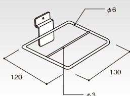
(P-U新) クロームメッキ シューズフック HP-SSHK コードNo. 定 価 55138 ¥1,680 梱30 185g
