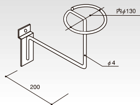
(P-小) クロームメッキ 帽子フック HP-HCHK コードNo. 定 価 55103 ¥2,170 梱30 122g
