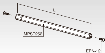
丸パイプセット クロームメッキ HP-MPST-585 L(mm) コードNo. 定 価 重さ(g) 585 55171 ¥1,710 392 885 55173 ¥2,110 590 棚20
