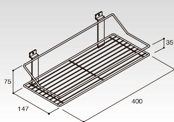
ミニバスケット (P-長) クロームメッキ HP-MBSK-N コードNo. 定 価 800g 55151 ¥8,030 棚5
