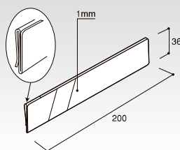
シューズフック用PCレール 透明塩ビ FU-PCR コードNo. 定 価 30g 55175 ¥820 ※FU型シューズフック専用 棚100
