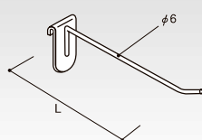
シングルフック φ6 HL-HK6-150 (棚50) (P-大) クロームメッキ L(mm) コードNo. 定 価 重さ(g) 150 62041 ¥630 84 200 62042 ¥660 95 250 62043 ¥730 107
