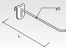
シングルフック φ5 HL-HK5-100 (棚100) (P-小) クロームメッキ L(mm) コードNo. 定 価 重さ(g) 100 62021 ¥500 37 150 62022 ¥560 46 200 62023 ¥600 51 250 62024 ¥660 59
