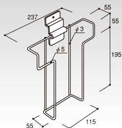
マガジンフック (P-U大) クロームメッキ HP-MZHK コードNo. 定 価 266g 55150 ¥3,450 棚15
