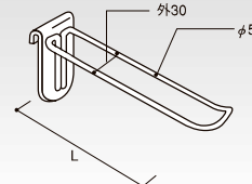
ダブルハンガー 巾30 HL-WHG30-150 (棚30) (P-大) クロームメッキ L(mm) コードNo. 定 価 重さ(g) 150 62051 ¥1,420 100 200 62052 ¥1,480 115 250 62053 ¥1,780 130
