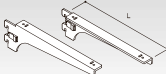
木棚ブラケット一体型(SP) (右・左セット) クロームメッキ NX443/L-R-120 SP L(mm) コードNo. 定 価 重さ(g) 120 76939 ¥1,050 280 170 76940 ¥1,170 320 220 76941 ¥1,300 390 ※ブラケット用サポートが必要です。
