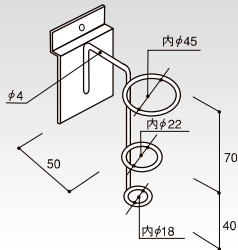
(P-大) クロームメッキ リングフック 3連 HP-R3HK コードNo. 定 価 55102 ¥3,750 梱30 145g
