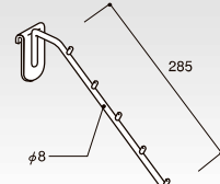
(P-大) クロームメッキ 傾斜フック HL-KSHK コードNo. 定 価 重(g) 195g 62091 ¥2,450 棚30
