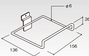
(P-U新) クロームメッキ FU型シューズフック HP-SSHK-FU コードNo. 定 価 55135 ¥2,100 梱30 197g
