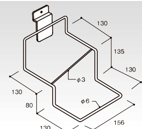
(P-U新) クロームメッキ シューズフック(2段/左傾斜) HP-SWHK/L コードNo. 定 価 55140 ¥2,240 梱15 320g
