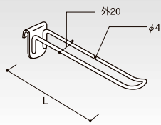
(P-小) クロームメッキ ダブルハンガー 巾20 HL-WHG20-100 コードNo. 定 価 重(g) 100 62055 ¥1,350 42 150 62056 ¥1,420 51 200 62057 ¥1,570 61 棚50
