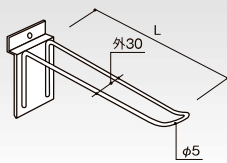
(P-中) クロームメッキ ダブルハンガー 巾30 HP-WHG30-150 L(mm) コードNo. 定 価 重さ(g) 150 55086 ¥1,340 125 200 55087 ¥1,410 141 250 55088 ¥1,800 156 梱30
