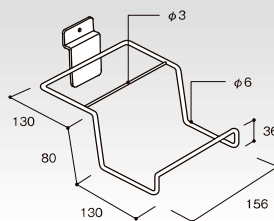
(P-U新) クロームメッキ FU型シューズフック(2段) HP-SWHK-FU コードNo. 定 価 55136 ¥2,170 梱15 300g
