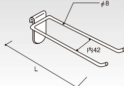
(P-大) クロームメッキ ダブルフック HL-WHK-200 コードNo. 定 価 重(g) 200 62061 ¥1,520 225 250 62062 ¥1,710 255 棚30
