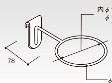
(P-大) クロームメッキ リングフック HL-115RHK コードNo. 定 価 重(g) 115 62085 ¥2,550 102 150 62086 ¥2,620 170 棚30
