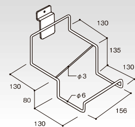
(P-U新) クロームメッキ FU型シューズフック(2段/左傾斜) HP-SWHK/L-FU コードNo. 定 価 55137 ¥2,280 梱15 330g
