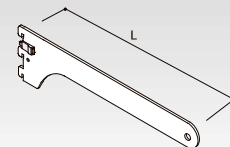
水平丸パイプ ブラケットBタイプ(SP) クロームメッキ NX523B-200 SP L(mm) コードNo. 定 価 重さ(g) 200 81872 ¥710 200 250 81873 ¥780 250 300 81874 ¥840 300 ※ブラケット用サポートが必要です。
