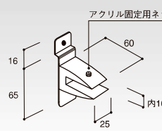
アクリル棚用ブラケット (P-専) クロームメッキ HP-ACBK コードNo. 定 価 100g 55174 ¥3,510 棚50
