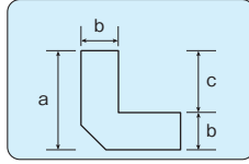
〈断面図〉 NC40、25
