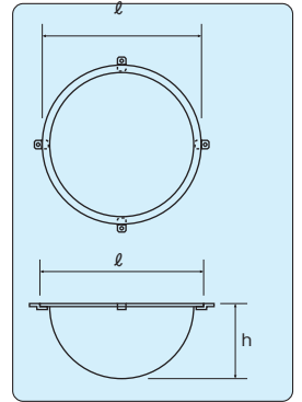
〈取付け図〉
