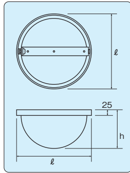
〈取付け図〉
