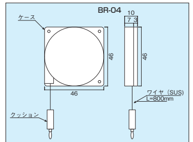
〈構造図〉
