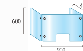
アクリルパーテーション三面タイプ窓付 APT3F-M600×900×450 27,000円(税抜) ※開口部H200×W300
