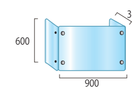
アクリルパーテーション三面タイプ APT3F600×900×300 23,000円(税抜)
