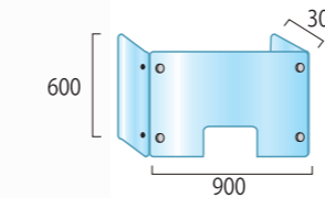
●アクリル板(透明)=厚さ3mm~4mm(※サイズにより異なります) ●金具=アルミ押し出し/アルマイト仕上(シルバー)
