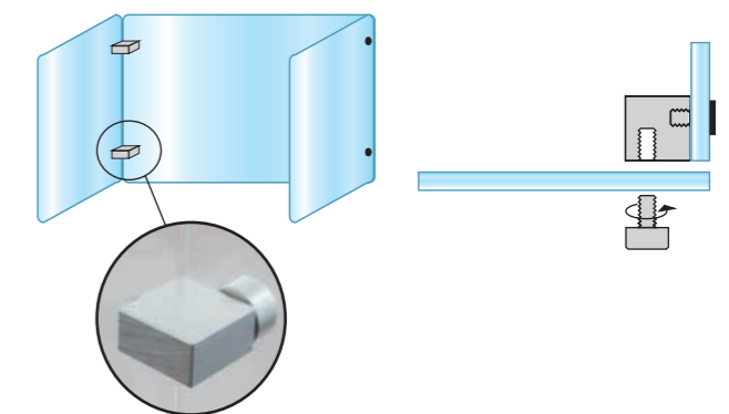
●アクリル板(透明)=厚さ3mm~4mm(※サイズにより異なります) ●金具=アルミ押し出し/アルマイト仕上(シルバー)
