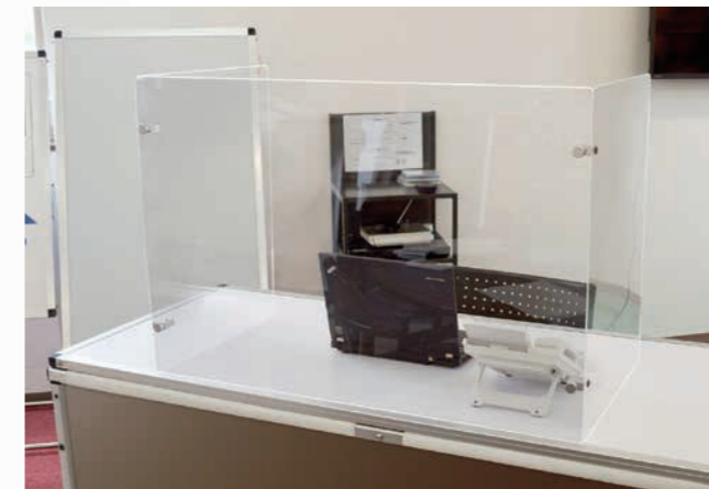
●アクリル板(透明)=厚さ3mm~4mm(※サイズにより異なります) ●金具=アルミ押し出し/アルマイト仕上(シルバー)
