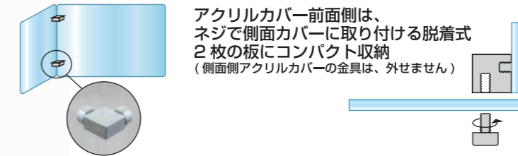
●アクリル板(透明)=厚さ3mm~4mm(※サイズにより異なります) ●金具=アルミ押し出し/アルマイト仕上(シルバー)
