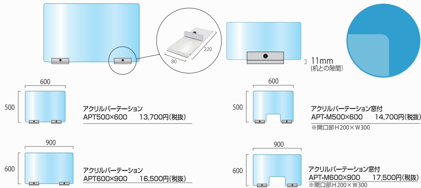
●アクリル板(透明)=厚さ3mm~4mm (※サイズにより異なります) ●ベース部=材質:スチール鋼鉄(SPHC) 表面処理:焼付け塗装(白色)
