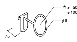
垂直リングフック
