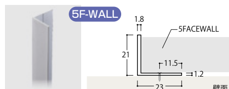
RH-CO コーナーレール
