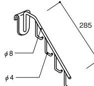
袋物フック HL-FHK
