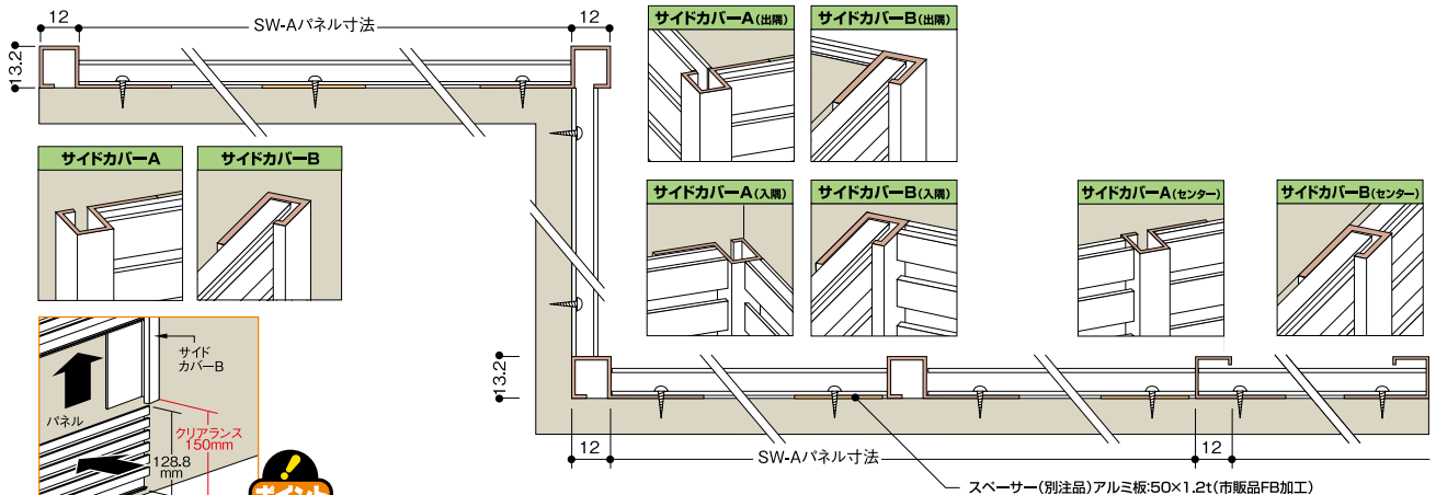
【水平断面図】
