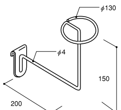
帽子フック HL-HCHK
