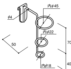
リングフック 3連
