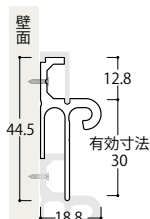
RH-SUB サブパネル
