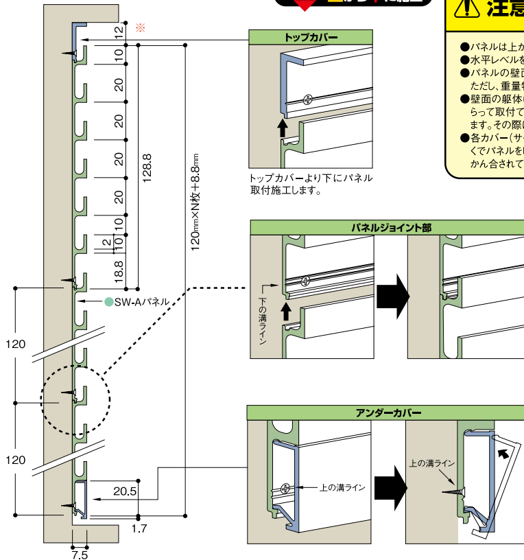
【垂直断面図】
