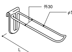
ダブルハンガー 巾30
