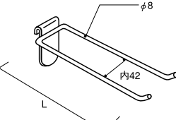
ダブルフック
