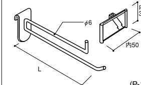
PCフック(カード差し付)
