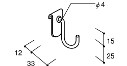
U型フック HL-UHK
