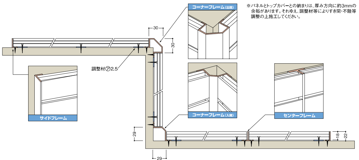
【水平断面図】
