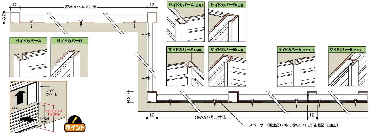
【水平断面図】
