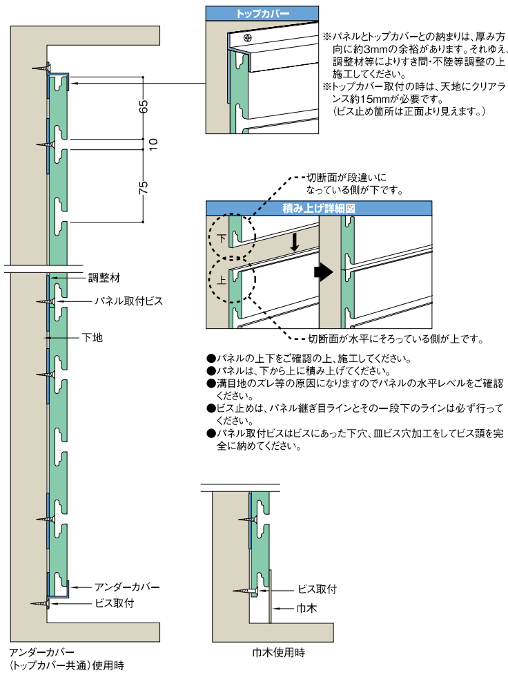
【垂直断面図】
