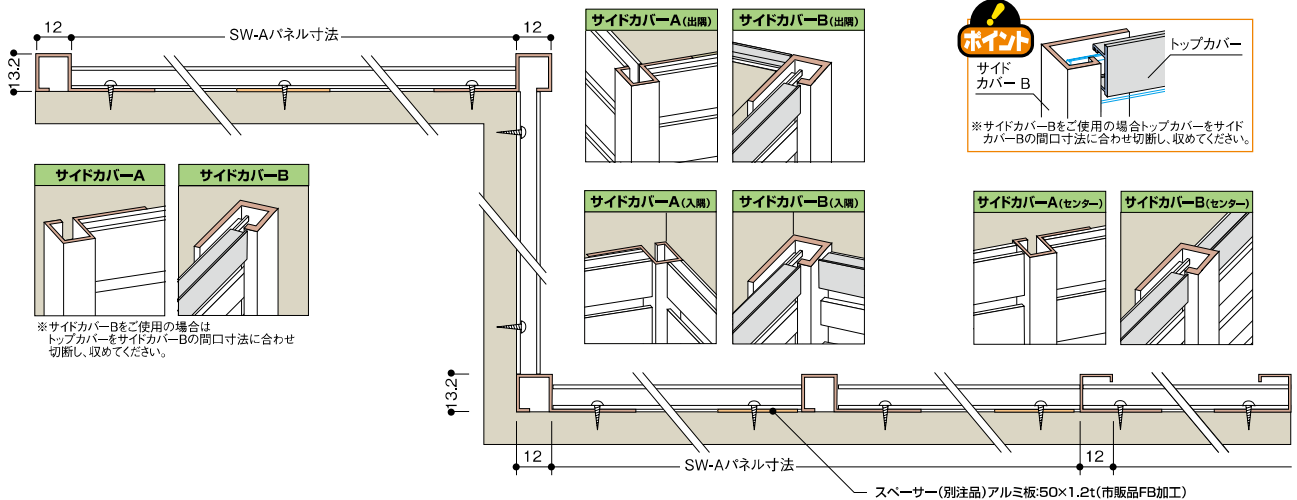
【水平断面図】
