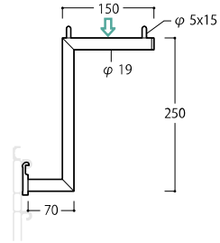
RH-UH アップハンガーフック
