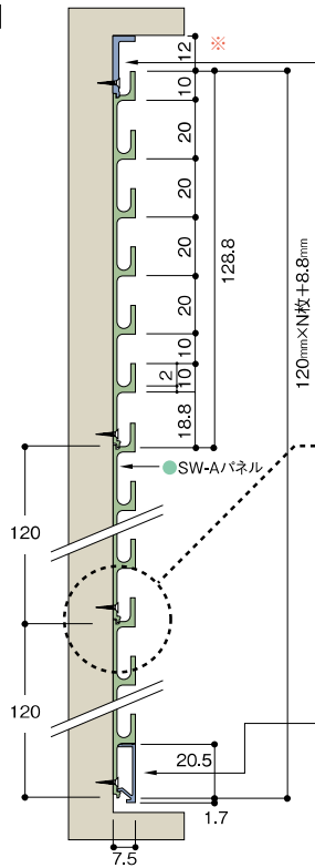
【垂直断面図】
