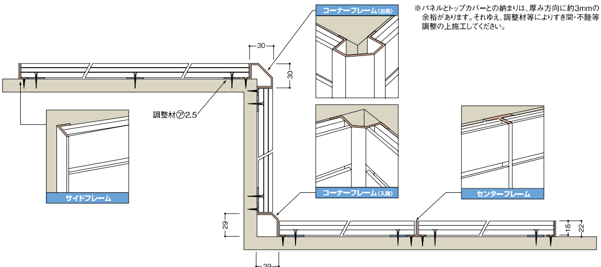
【水平断面図】
