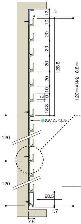
【垂直断面図】
