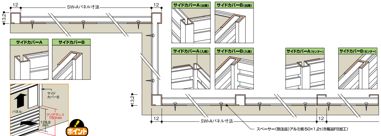
【水平断面図】
