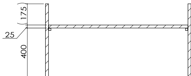
断面図 A-A ( S = 1 : 15 )
