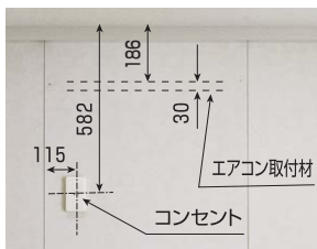
単位(mm)
