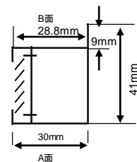
アルミフレームの断面図
