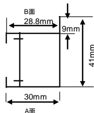
アルミフレームの断面図
