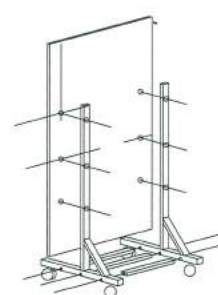
LA-11 組立図
