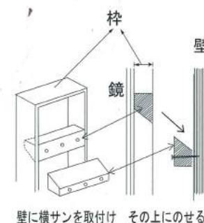
ドック式取付方法
