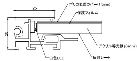
フレーム断面図
